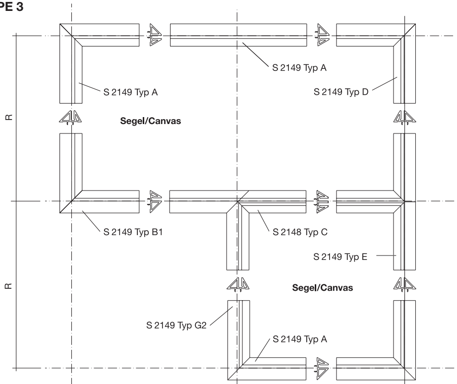
Profil 2149
