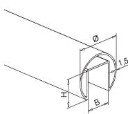
Ø 42,4 L 6000 mm AISI 304 B H 09.13.6920.042.12 24 24 Ø 48,3 L 6000 mm AISI 316 09.14.6920.042.12 24 24 Ø 60,3 L 6000 mm
