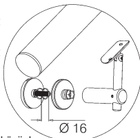
AISI 304 09.13.0155.000.12 AISI 316 09.14.0155.000.12
